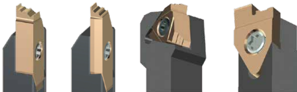
成型刀片 profiling inserts
